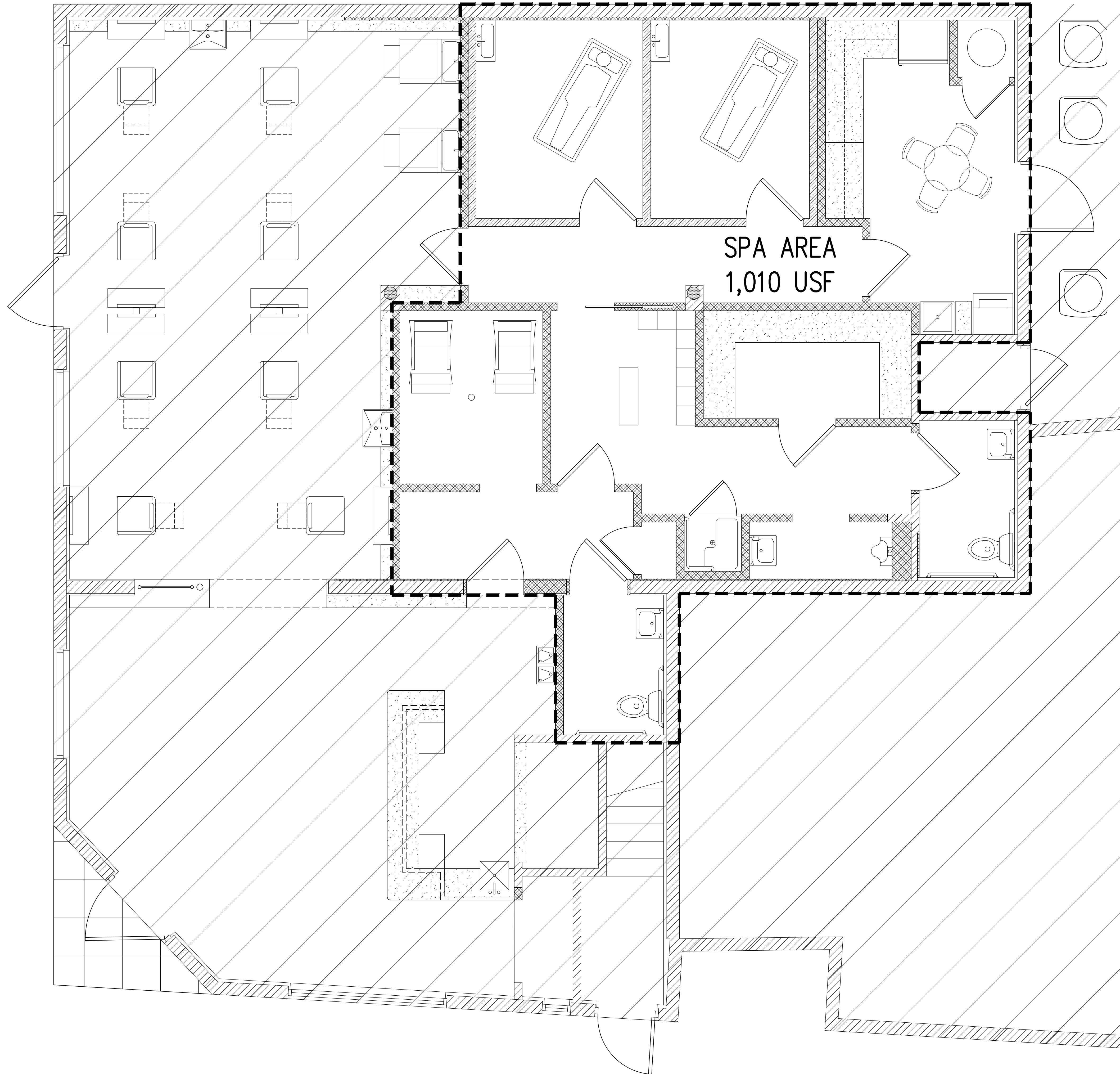
AREA PLAN SCALE: 3/8"=1'-0"
