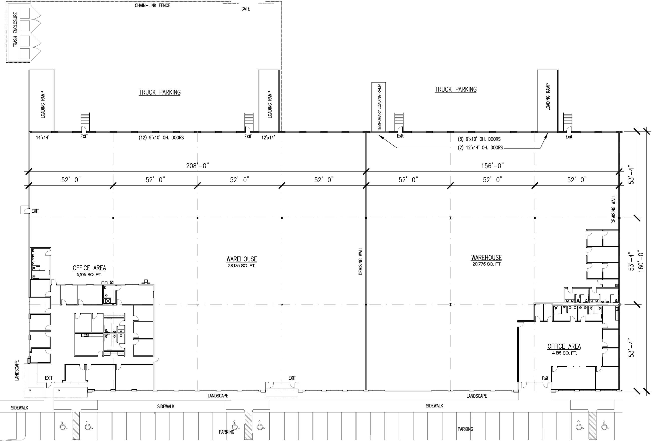
SUITE 100-200 FLOOR PLAN
